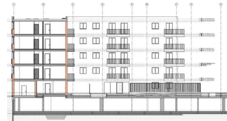
SECTION 01
